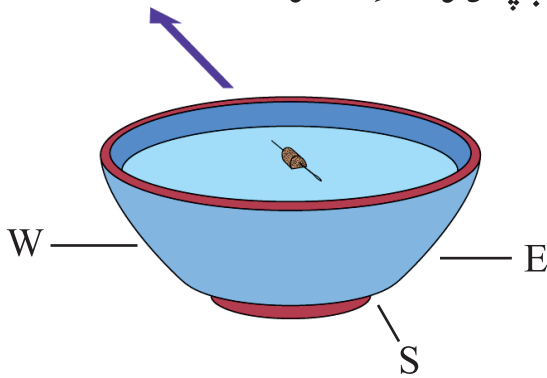
19.3: مقناطیسی سوئی
